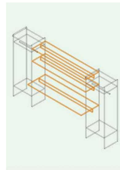
02-クローゼットにシェルフとデスクを固定
